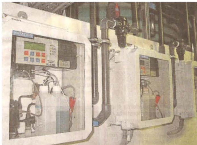
En sous-sol, des capteurs vérifient la composition chimique de l'eau et la modifient s'il le faut.
